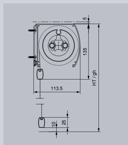
Soloroll® Box 105 sin guía
