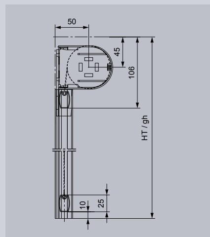
Soloroll® cojinete 80 rieles guía Fix
