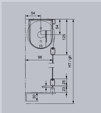
Soloroll® cojinete 100 guía por cable de enrollamiento exterior
