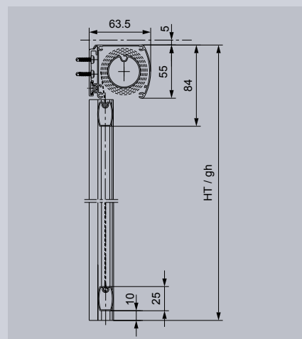
Soloroll® Box 55 rieles guía
