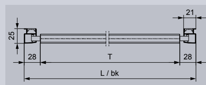
Soloroll® Box 105 sin guía
